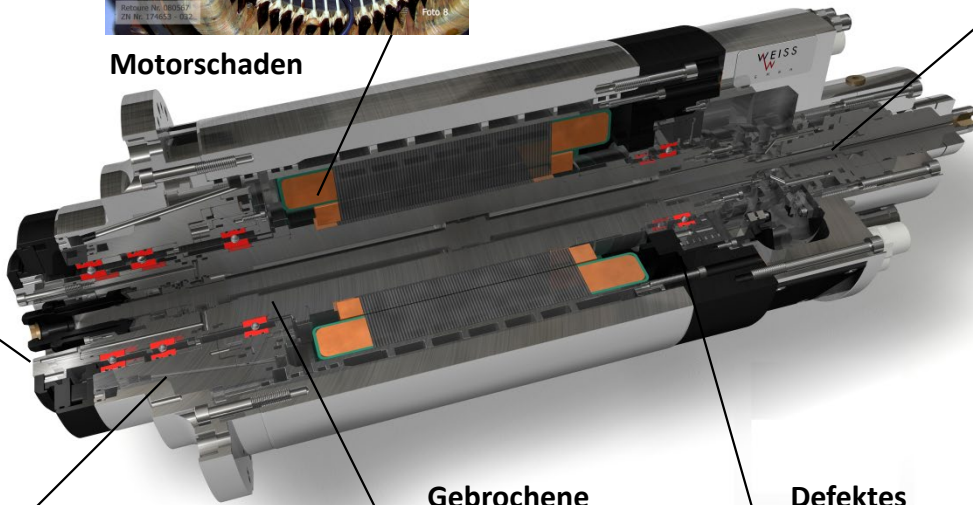
Defektes Festlager
