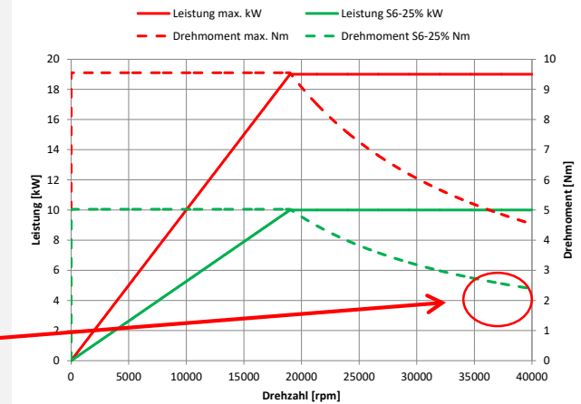
Motor Kennlinie
